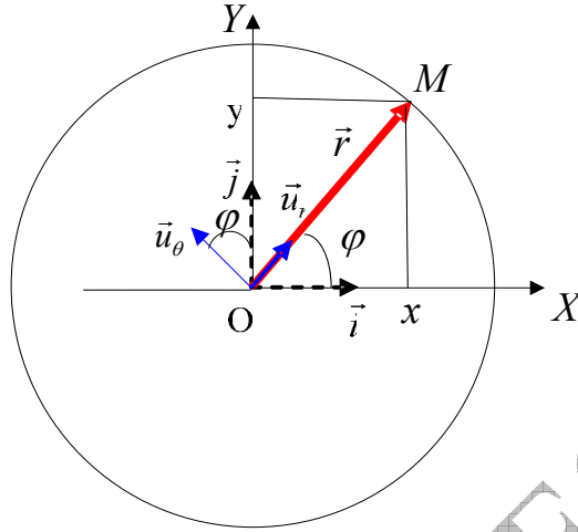
Fig 3.4: Coordonnée polaires
